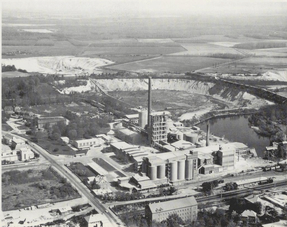
Oben: Die Portland-Zement-Fabrik in Misburg. Der Blick von oben zeigt das Industriewerk vor den Abbau-Anlagen und der Seen-Bildung. Portland-Schichten, das sind Kalke, Tone, Mergel und Oolithe, die sich zur Zementfabrikation eignen.
