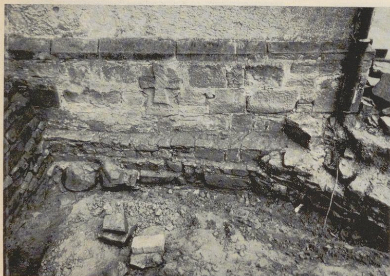
Abb. 6 Frühgotische Quadergrundmauer der Westwand des Südschiffes; darauf aufsetzend die hochgotische Westwand (mit eingemauertem Kreuzstein)
